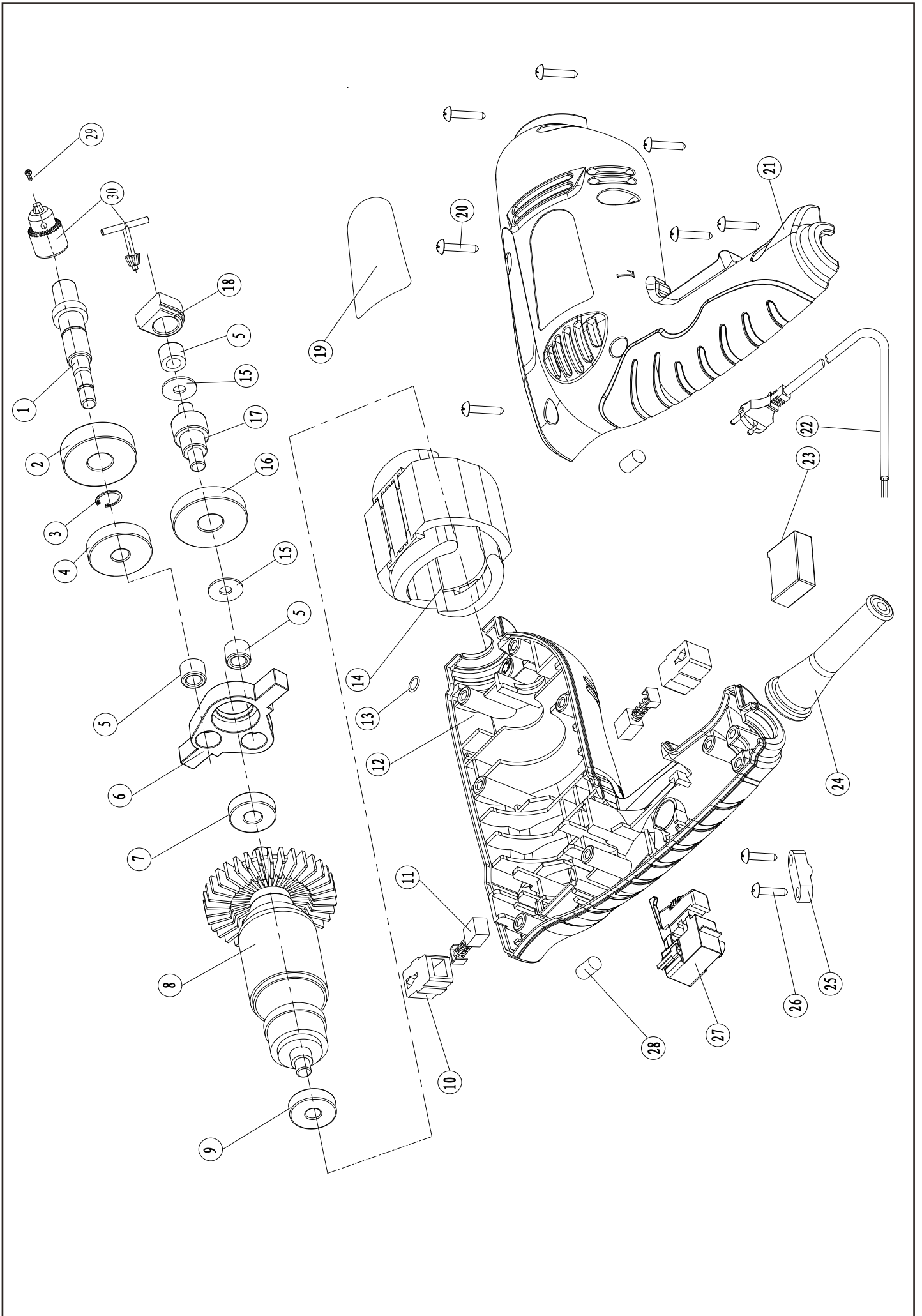
D103RE电钻爆炸图
