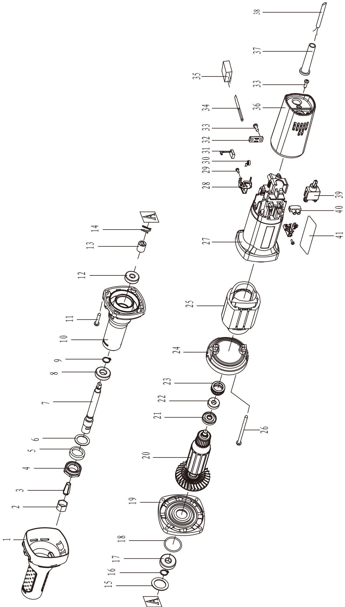
DG30电磨爆炸图
