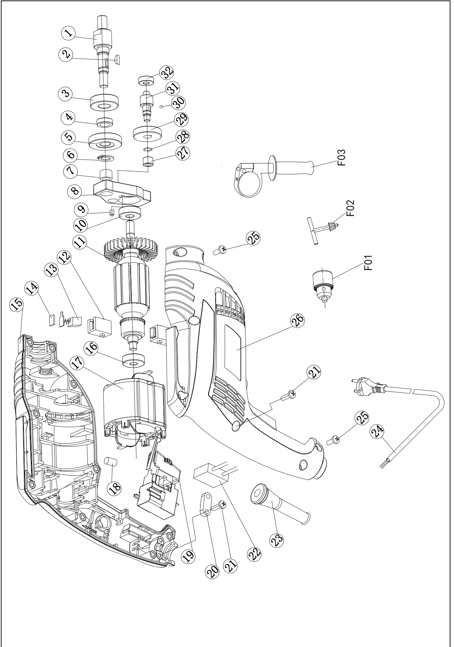
D13RE电钻爆炸图
